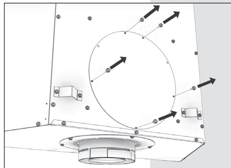
Retirez les cinq (5) vis no 10AX1/2 HX qui fixent la plaque de couverture à l'arrière du foyer.
