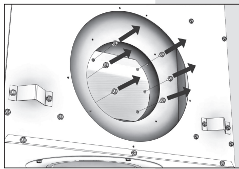
Retirez les six (6) vis no 10AX1/2 HX qui fixent l'obturateur d'échappement à la boîte à combustion.
