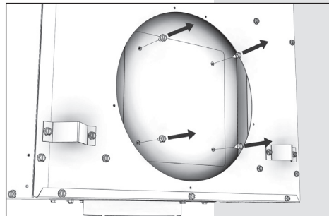
Retirez les quatre (4) vis no 10AX1/2 HX qui fixent la plaque de couverture à la chambre d'admission.
