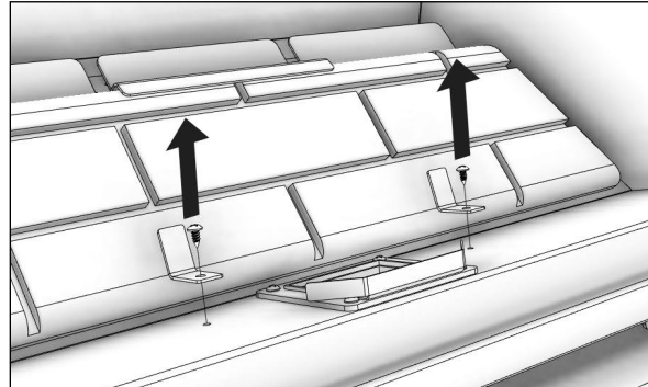
Retirez les deux supports du panneau central.
